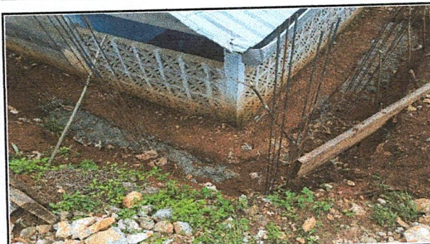
Foto 16: Reparación de muro de contención
